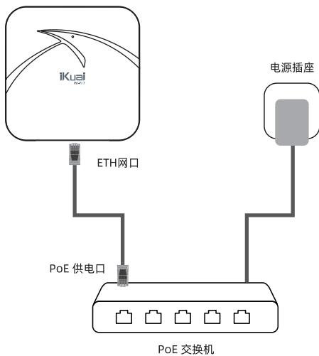
AP配置
